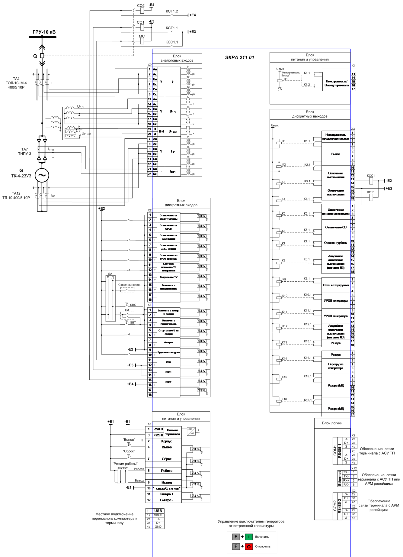
Рисунок 53 – Пример подключения внешних цепей к терминалу защиты генератора
