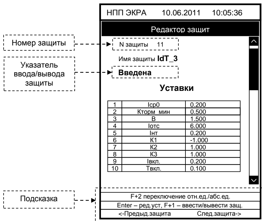
Рисунок 3 – Внешний вид меню Редактор защит
