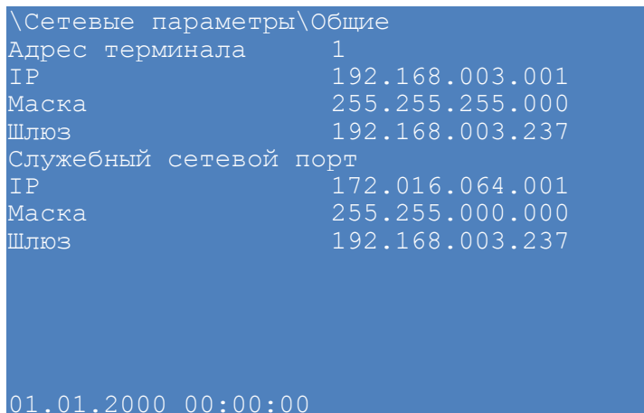
Рисунок 27 – Внешний вид подменю Общие
