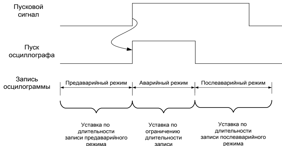
Рисунок 6 – Диаграмма формирования осциллограммы при длительном пусковом сигнале
