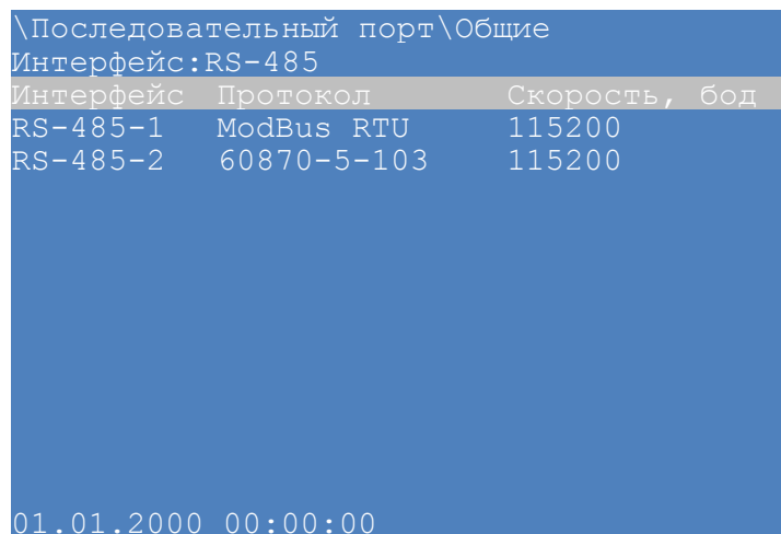
Рисунок 28 – Внешний вид подменю Общие
