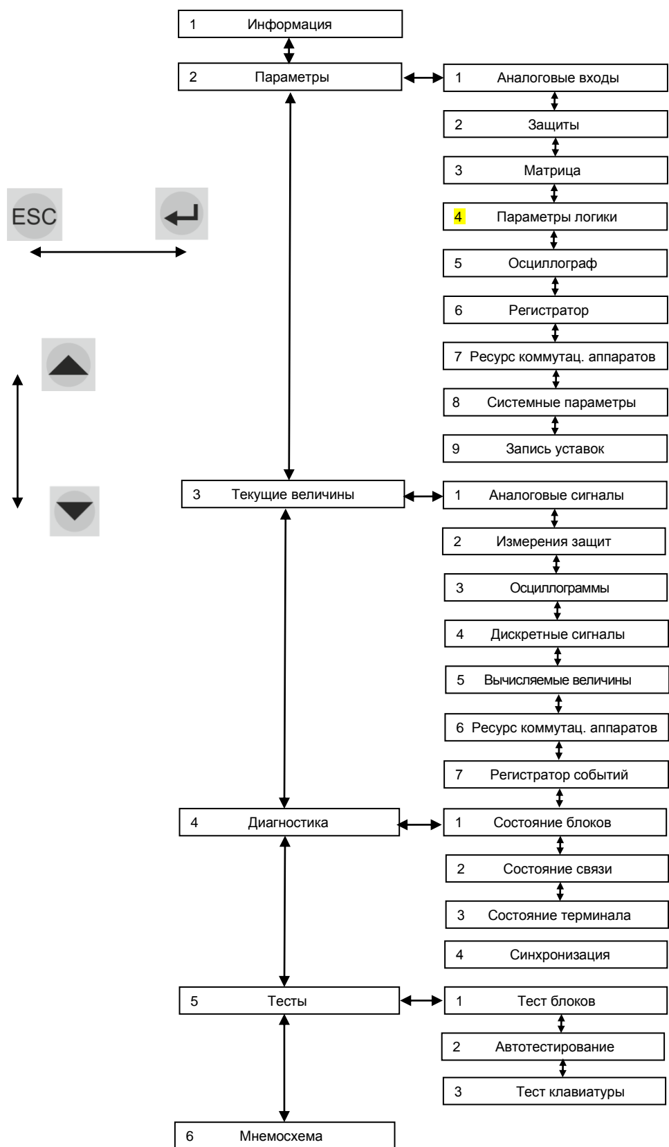
Рисунок 14 – Структура меню терминала с горизонтальным расположением дисплея
