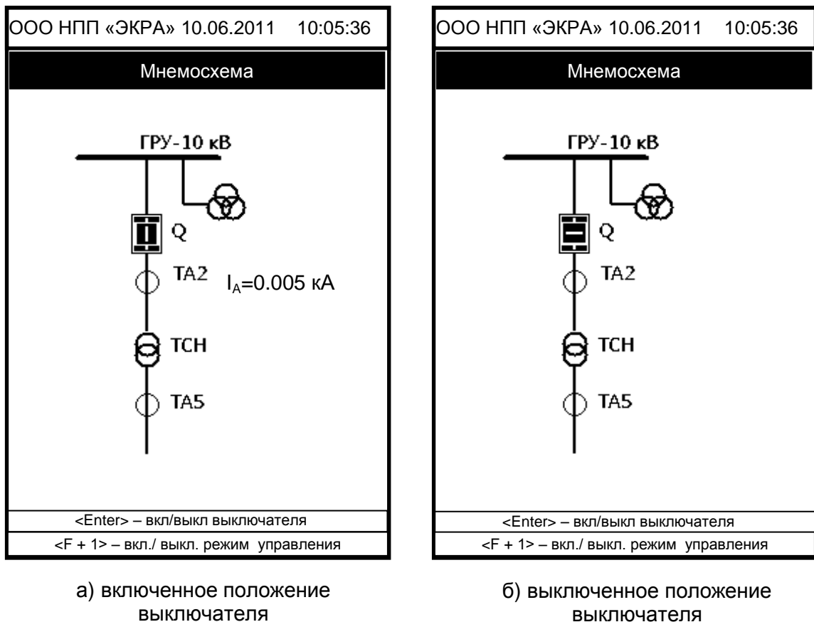
Рисунок 13 – Внешний вид пункта меню Мнемосхема
